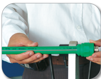
Bước 5: Nối các bộ phận cần hàn với nhau, không được xoay trong lúc nối Joint the pipe & the fitting by pushing the pipe until it reaches the mark, both parts must remain fixed, without rotation during the joining time
